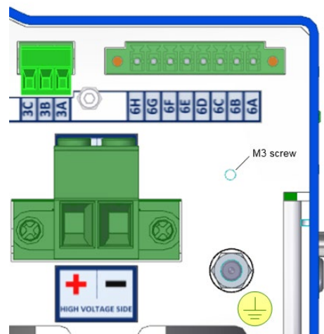
Fig. 8 EPC connector 6
