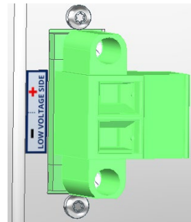
Fig. 6 LVDC link Size 3
